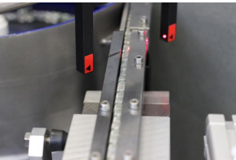
Linearförderstrecke
